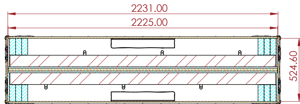
SECTION A-A SCALE 1 : 18
