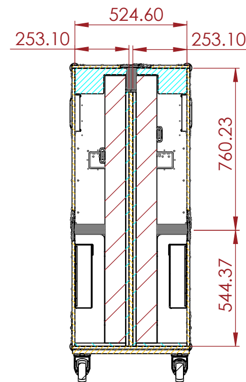
SECTION B-B SCALE 1 : 18
