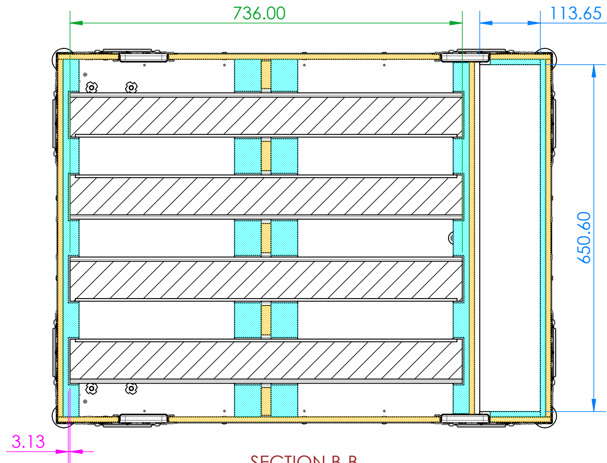
SECTION B-B SCALE 1 : 7
